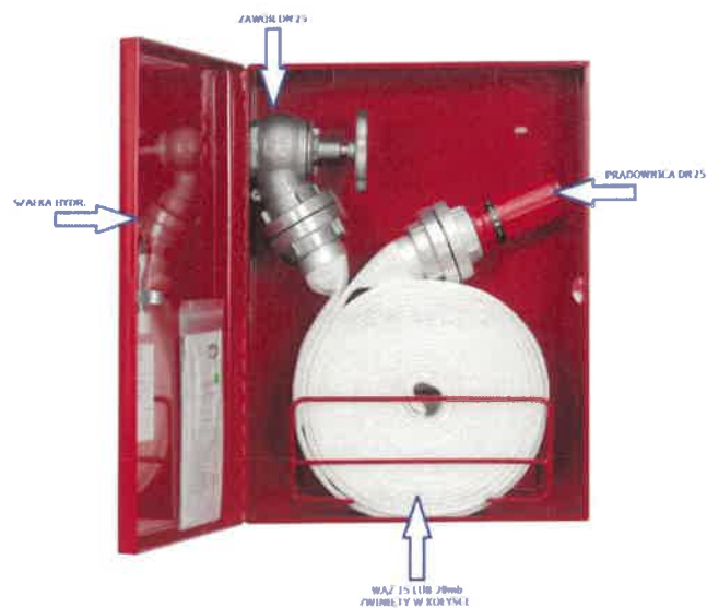
Hydrant z węzłem płasko składanym
