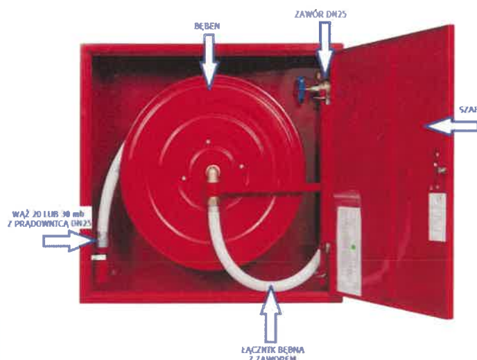
Hydrant z węzłem półsztywnym
